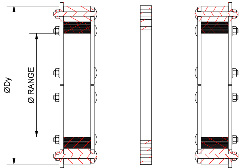
A-A ( 1 : 5 )
